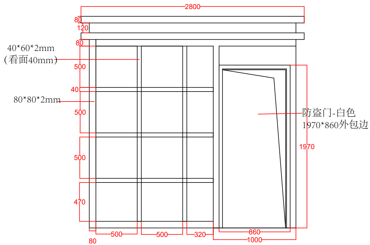
左侧骨架图
