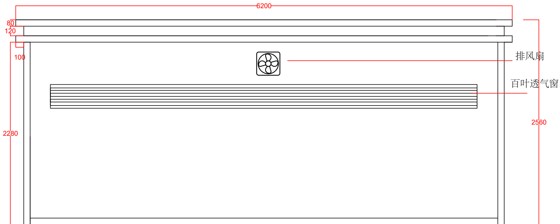
背面图
