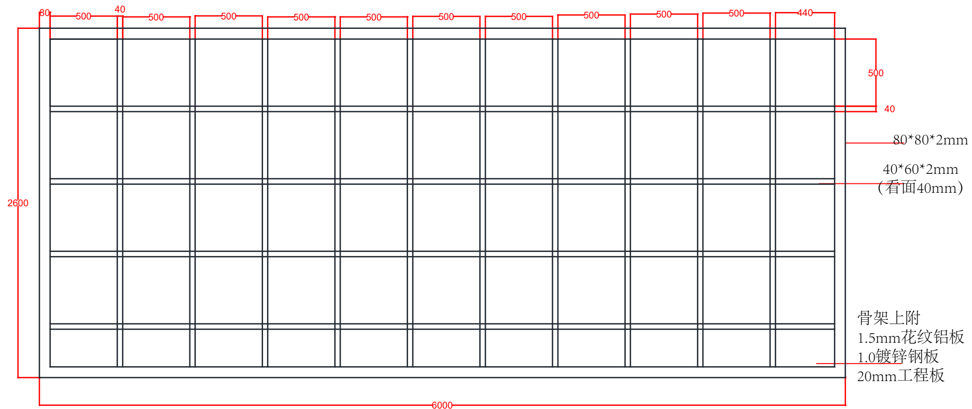
底部骨架图
